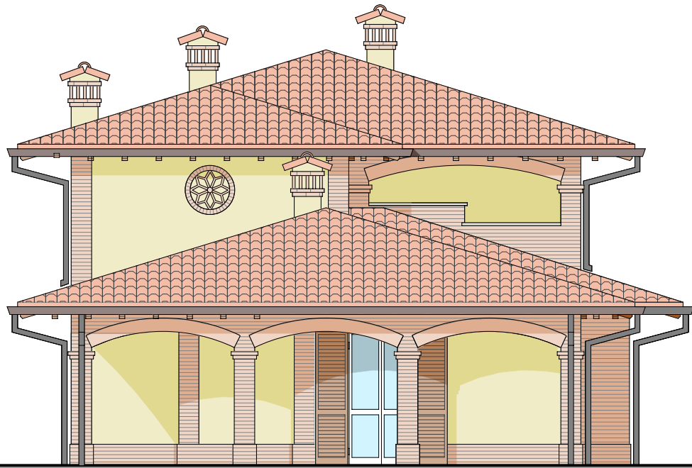
PROSPETTO NORD
